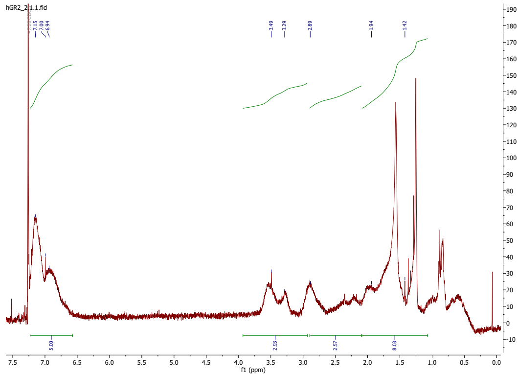
Abb. 17: NMR-Spektrum der Polystyrol- co -Polymethylmethacrylatprobe nach der Fällung.
